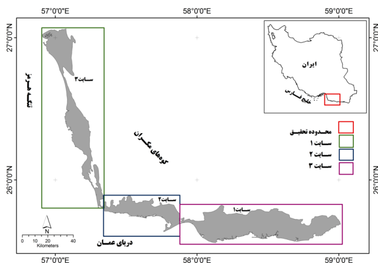
شکل ۲. تفکیک سایت‌های اصلی منطقه پژوهش
