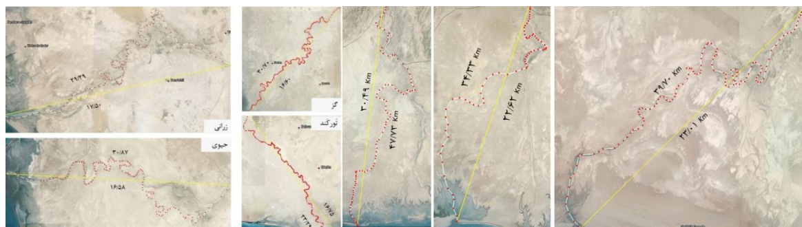
شکل ۶. سینوسیته رودخانه‌های منطقه؛ راست به چپ: تورکند، گز، حیوی، زرانی، سدیح، گابریک و جگین
