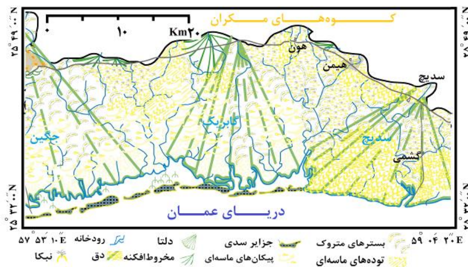
شکل ۵. مقطعی از نقشه ژئومورفولوژی منطقه دربرگیرنده دلتاهای سدیج، گابریک و جگین
