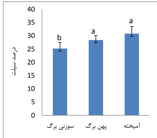
شکل ۵. مقایسه درصد سیلت خاک در توده های پهن برگ، سوزنی برگ و آمیخته در منطقه مورد تحقیق
