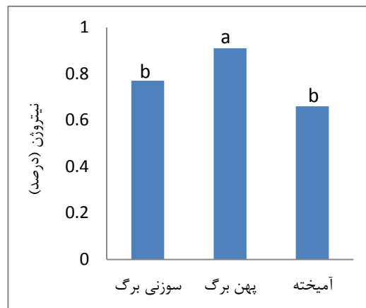
شکل ۹. مقایسه نیتروژن خاک در توده‌های پهن‌برگ، سوزنی‌برگ و آمیخته در منطقه مورد تحقیق
