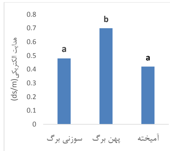
شکل ۳. مقایسه هدایت الکتریکی خاک در توده‌های پهن‌برگ، سوزنی‌برگ و آمیخته در منطقه مورد تحقیق
