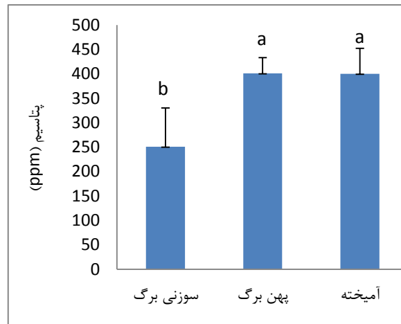
شکل ۷. مقایسه پتاسیم خاک (محللول و تبادل‌پذیر) در توده‌های پهن‌برگ، سوزنی‌برگ و آمیخته در منطقه مورد تحقیق
